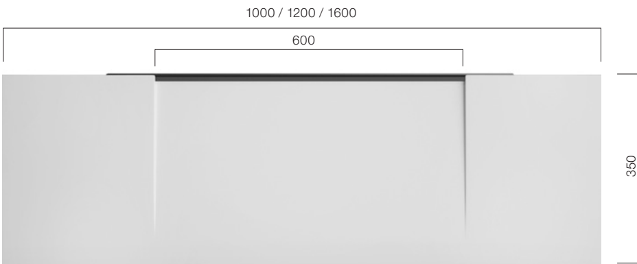
Tiefe der Ablauffläche: 80 mm; Waschtischhöhe: 40 mm
